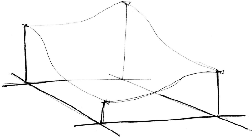
Cúbica (Hermite)
